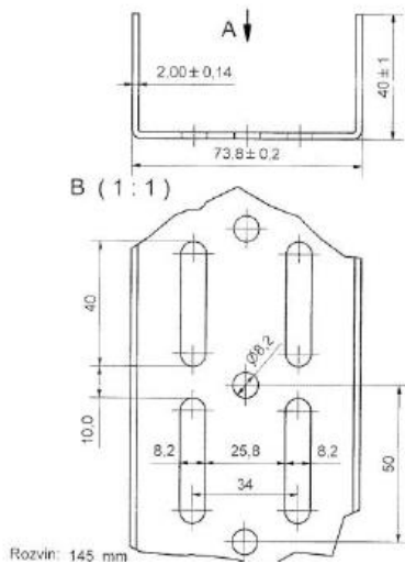
Profil UA 75
